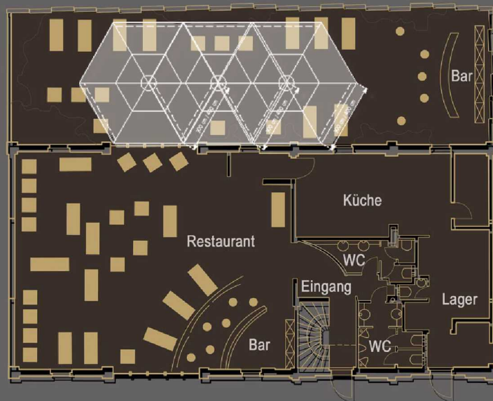
GRUNDRISS BASIL
